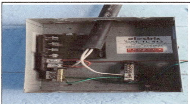
Foto 9: Sustitución de flípones. Modulo 1
